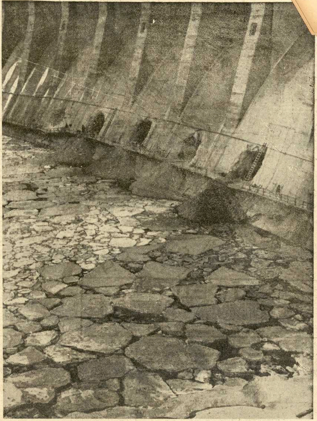
Кад је вода пуштана кроз тунел, снизио се ниво воде. Сваки тунел био је 25 квадратних метара величине, тако да је бреша остала на суву.
