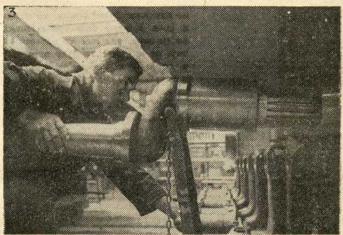
3 — Осовина главног точка који покреће гусеницу мора се „дихтовати“ да не пропушта ни кап воде кад тенк гази по води.
