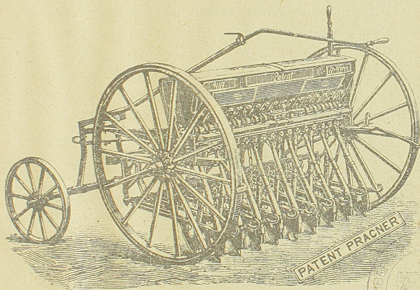
Машина за сејање „на врсте“ у 16 врста, тако звана „Будућност“.
