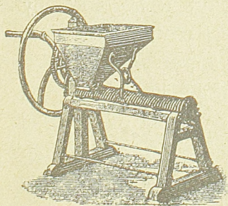
Машина за ломљење беја.
