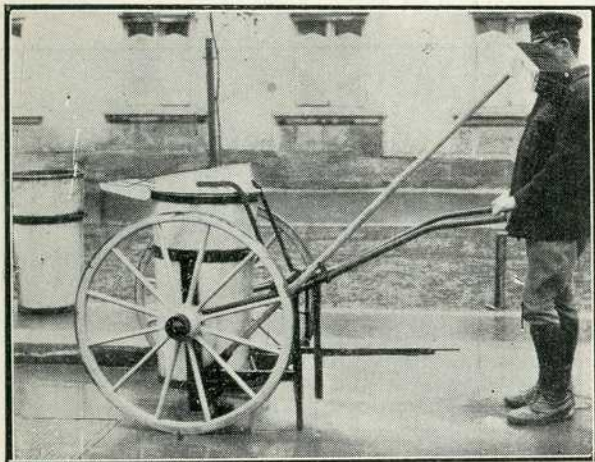
Сл. 5. — Поклопац — ђубравник затвара канту, сметлиште изручено у њу
