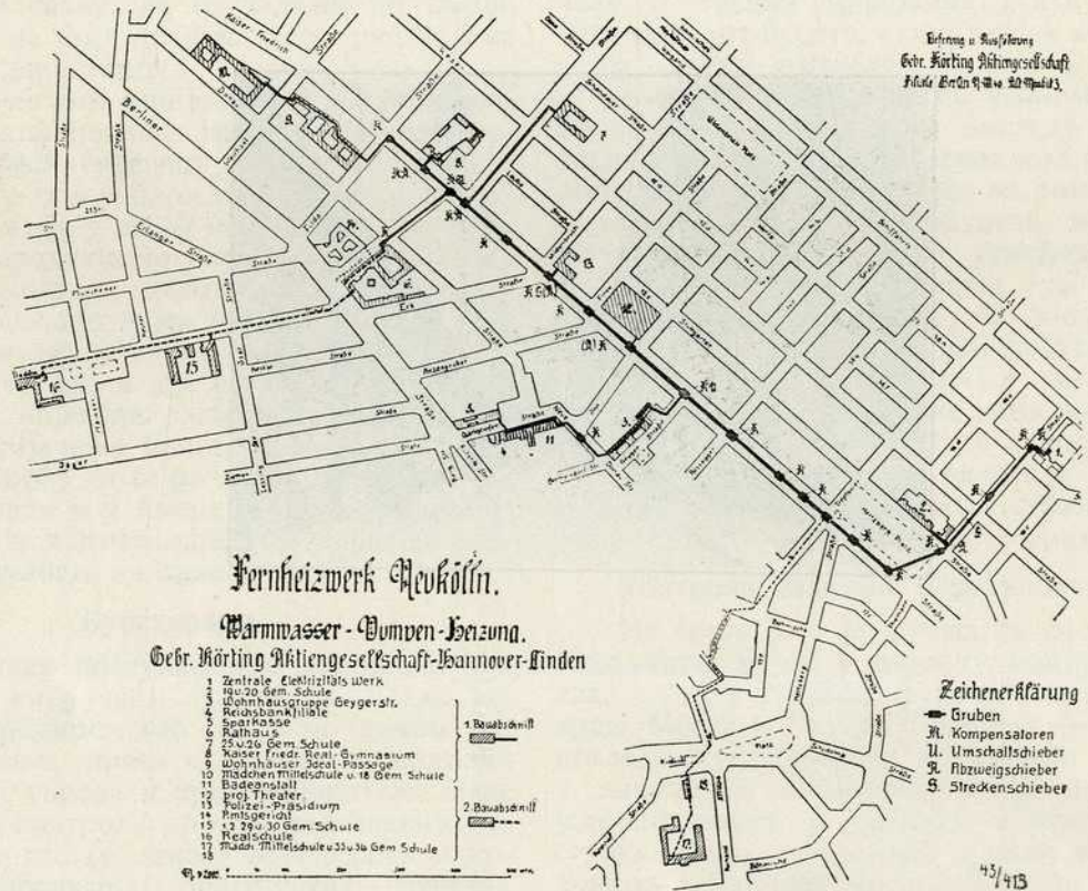
План мреже за грејање на даљину једног дела града (Берлин—Најкелн). При- кључци за поједине зграде означени су тачкама.
