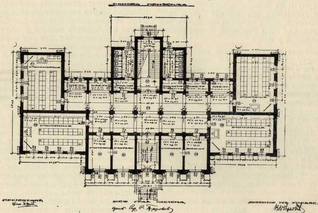
Основна школа у Булбулдеру. — Основа приземља
