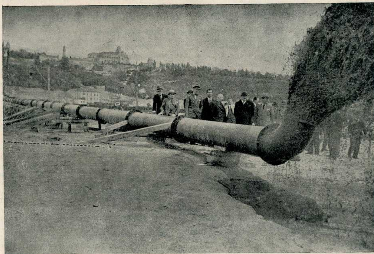
Почетак радова на насипању земљишта на левој обали Саве. Багер избацује огромне количине песка из речног корита
