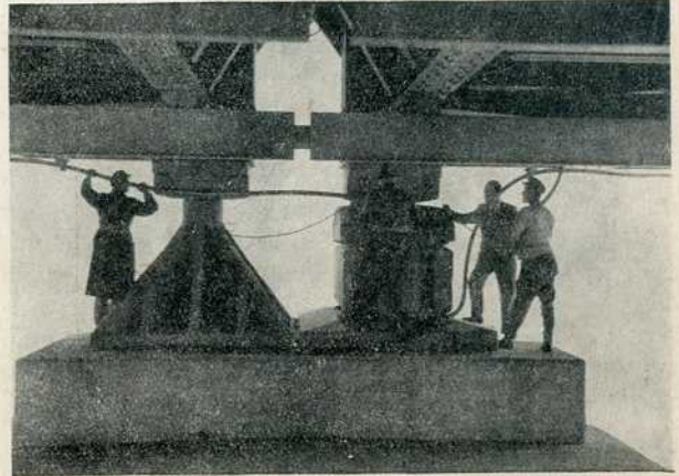
Полагање електричног кабла преко моста Краља Петра II.
