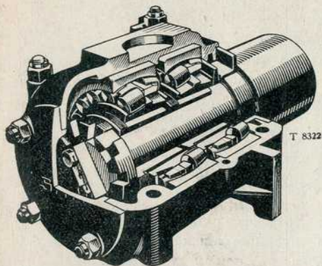
С К Ф МАЗАЛИЦЕ НА ВАЉКАСТИМ ЛЕЖАЈИМА.
