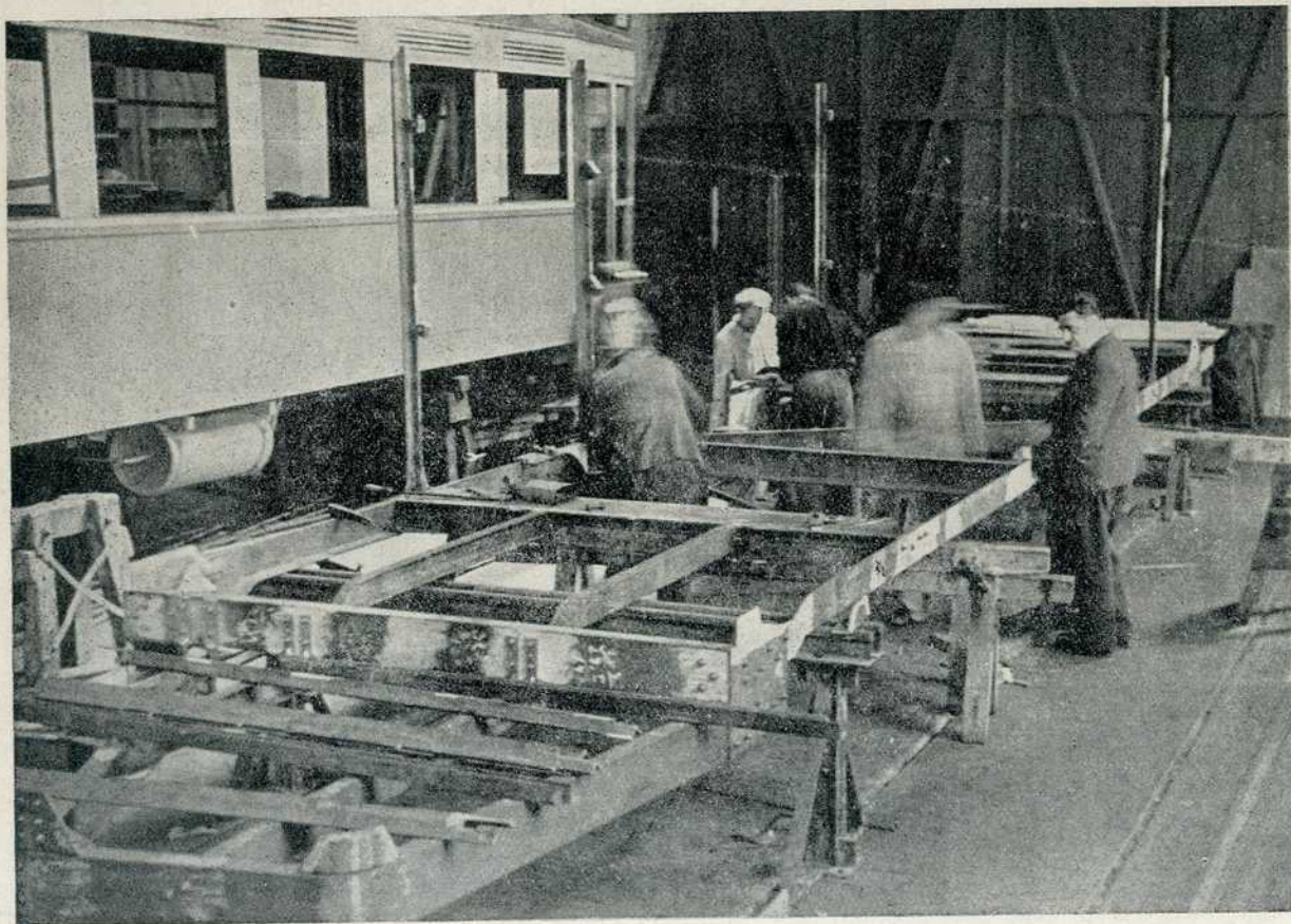
Грађење новог трамваја у радионици Д. Т. и О.
