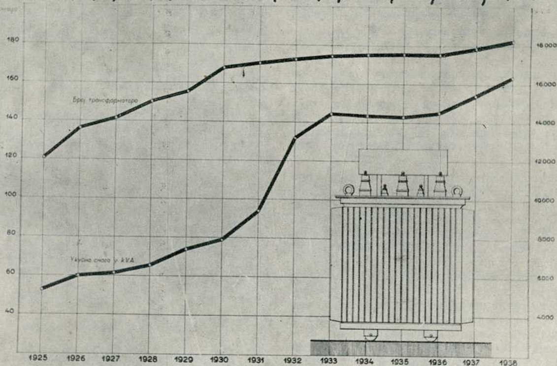
Развој броја и укупне снаге трансформатора од 1925 до 1938.
