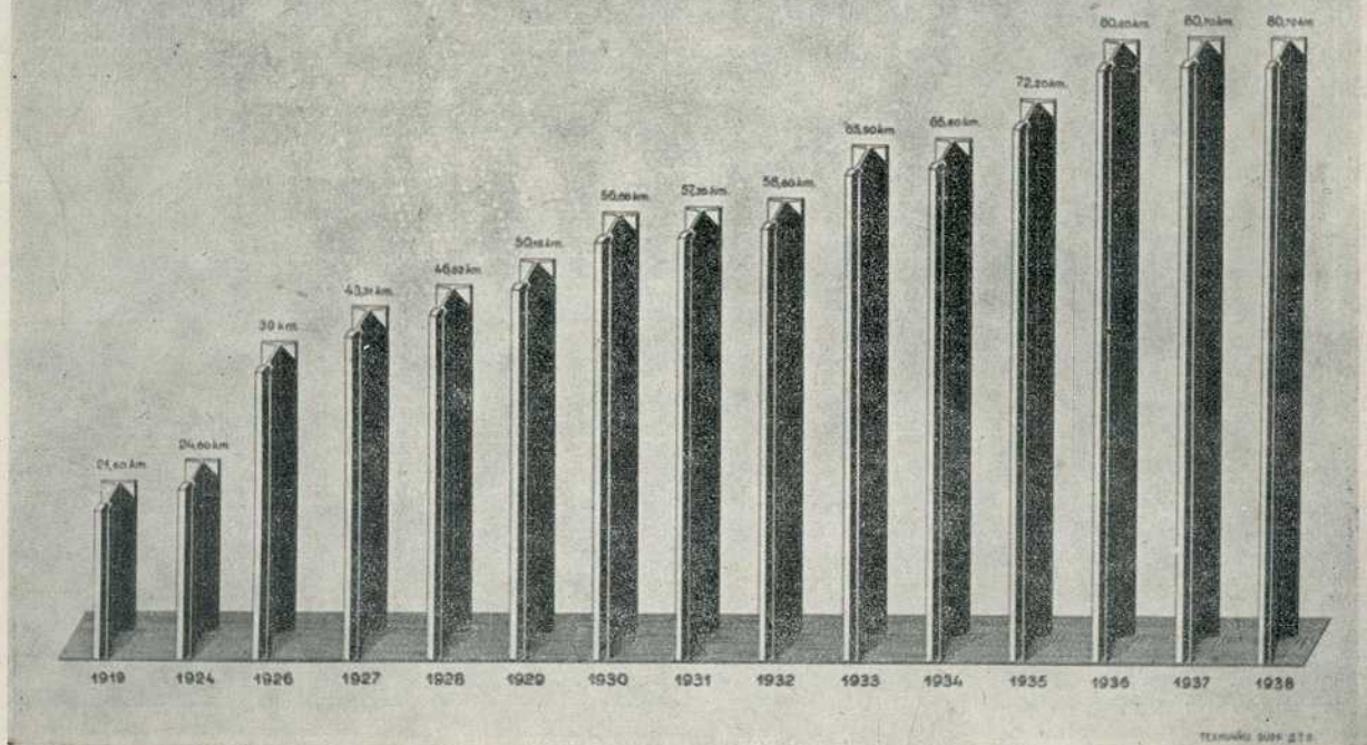
Грађевинска дужина трамвајских пруга у Београду у километрима
