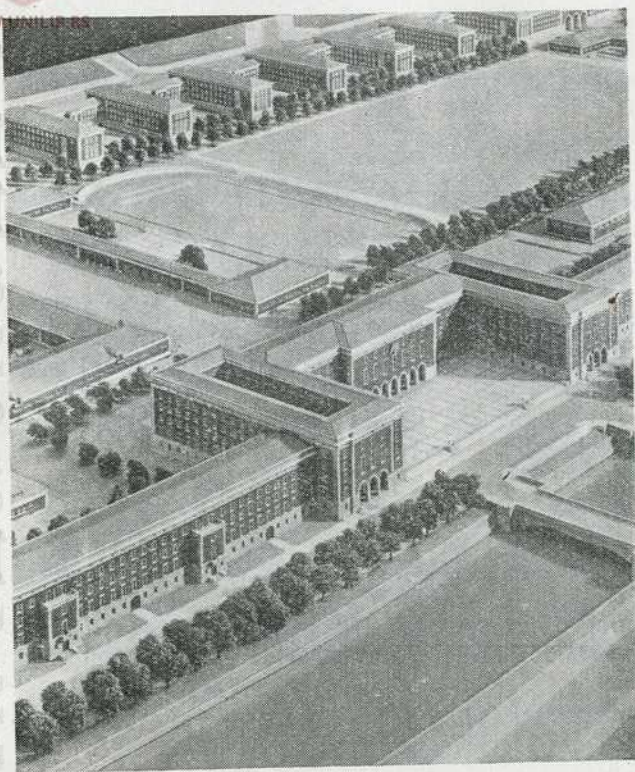
Архитект Ханс Херман Клаје, сарадник Ерих Фишке: Нове Касарне пука Велика Немачка у Берлину. Из пројектовања генералног грађевинског инспектора за главни град Рајха. Део модела
