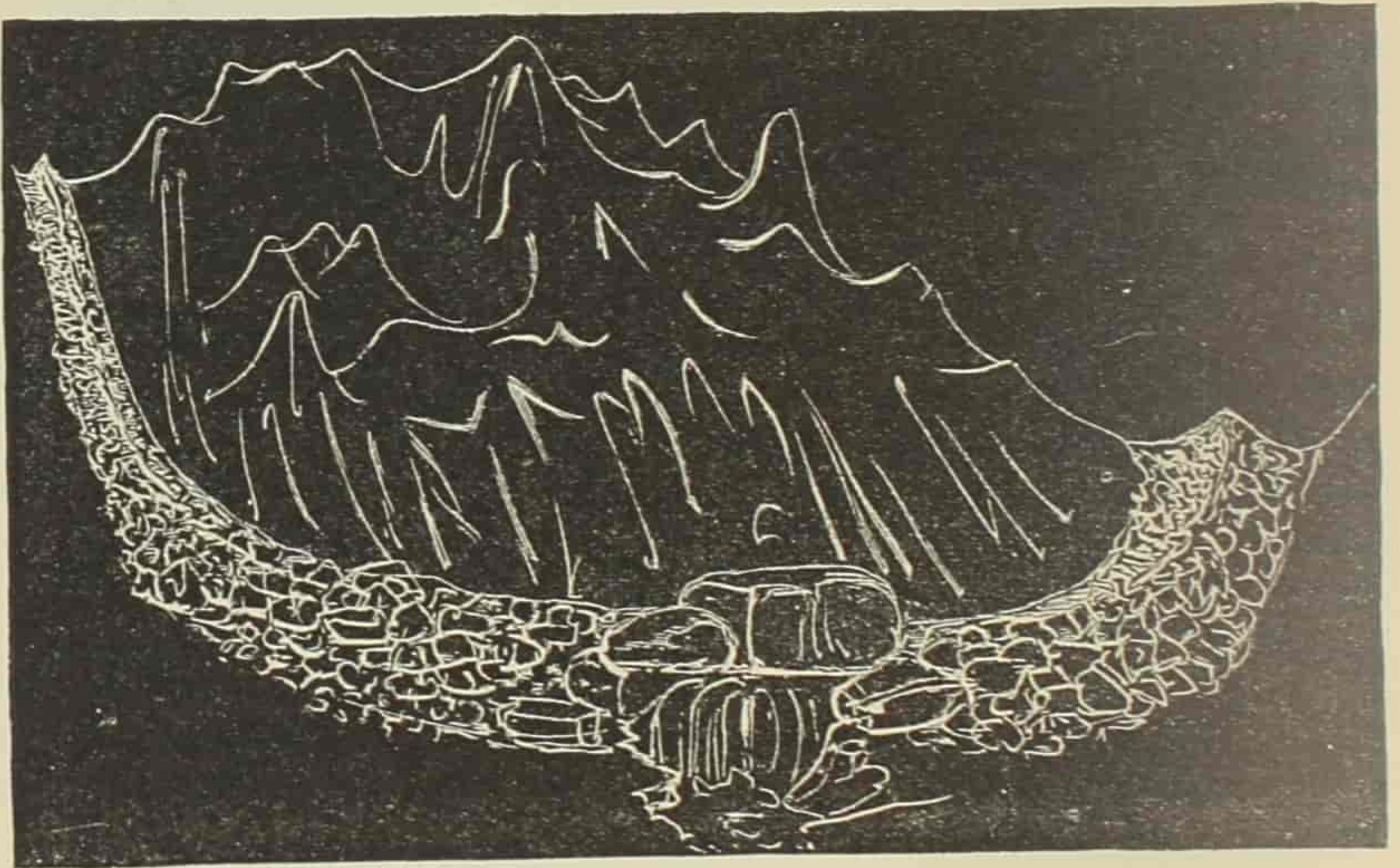
TERMINAL MORAINE.
